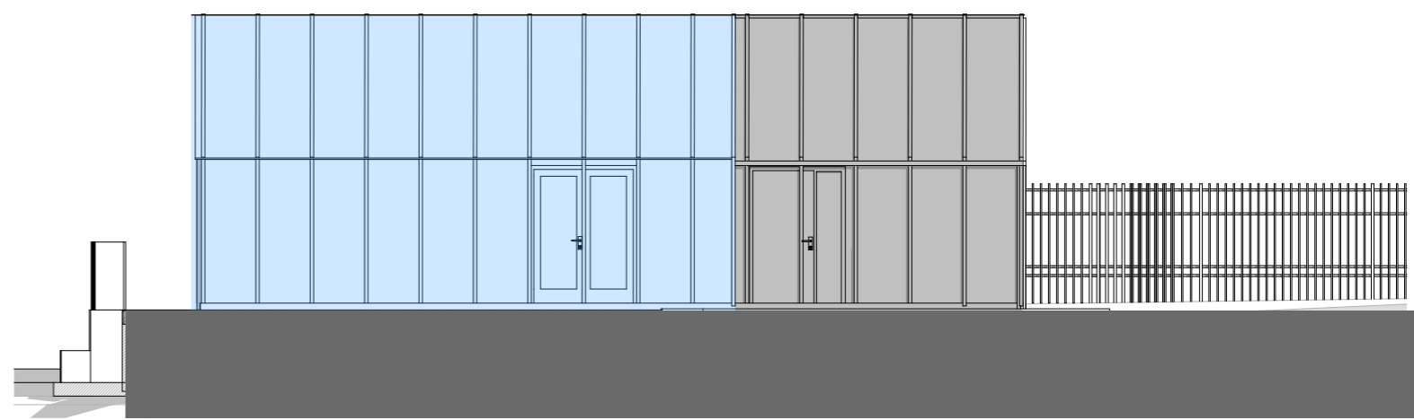
Fasade Ø
